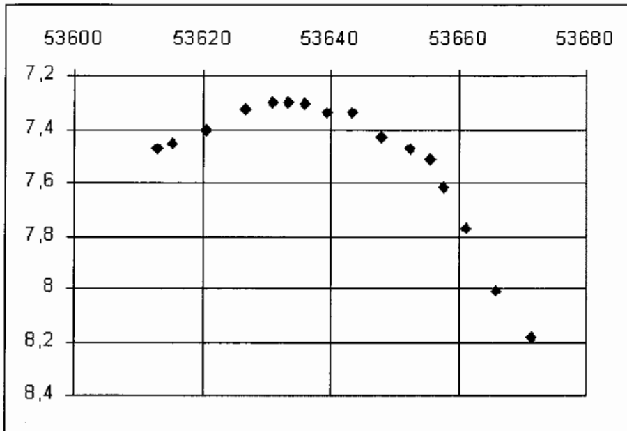
Courbe de lumière de R Dra
