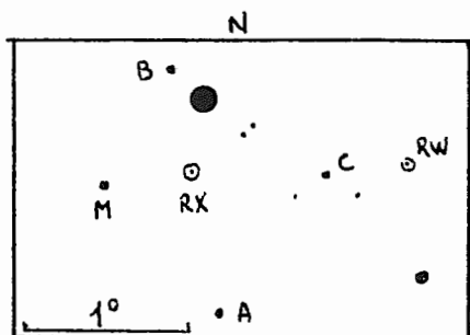
fig. 1 : Champ de RX Cam
