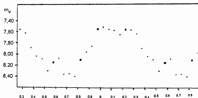
figure 3 : Courbe de lumière obtenue en calculant les moyennes par tranches de 0,05 phase. Les gros points correspondent aux moyennes d'au moins 5 observations.
